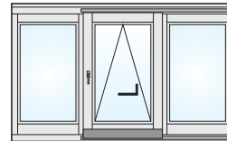
TYP 14 PSK-B Parallel Schiebekipptür einteilig, dreiflügelig
