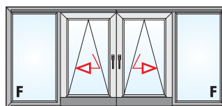
TIP 14R-C PSK drсна balkonska vrata enodelna - štirikrilna
